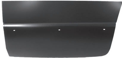
DOOR LWR SKIN: SLIDING DR ..... 1576-173L 38.125"W x 19"H
